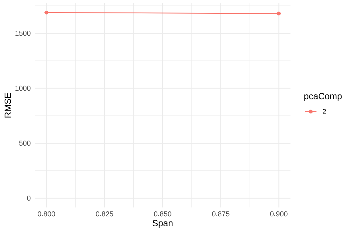
Lokaloji regresija: Kuko matas
