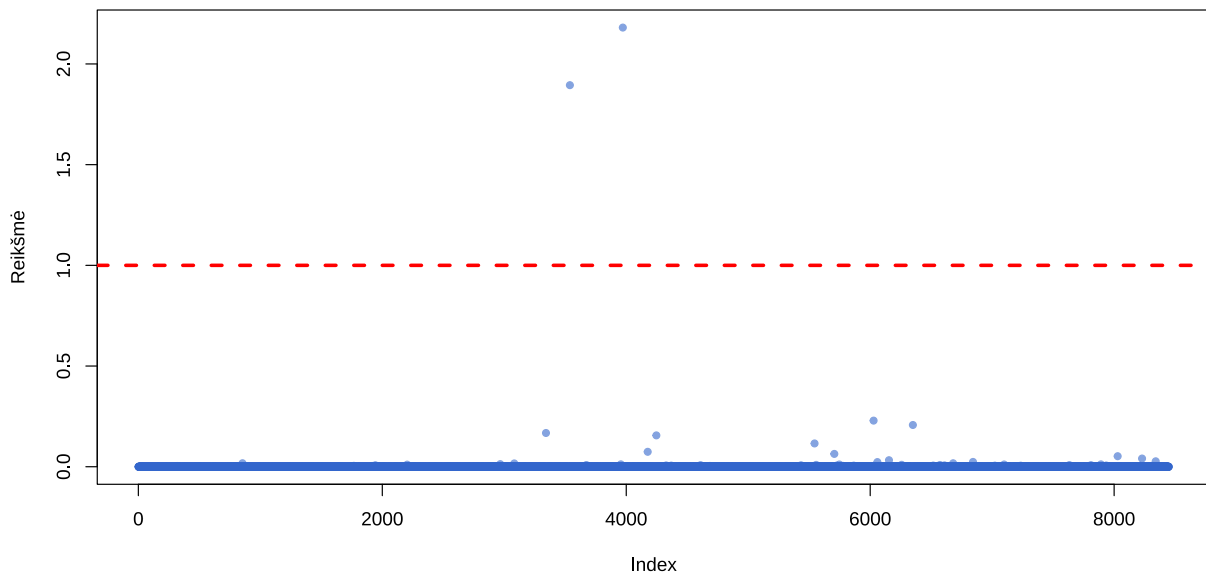
B-splinas: Kuko matas
