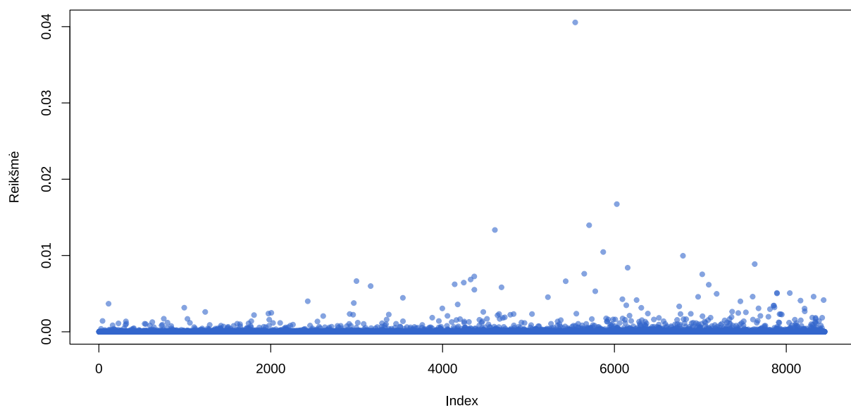
Lokaloji regresija: Kuko matas
