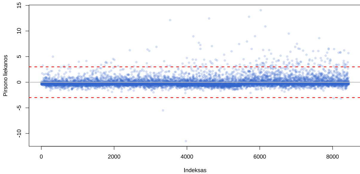
B-splinas: Pirsono liekanos
