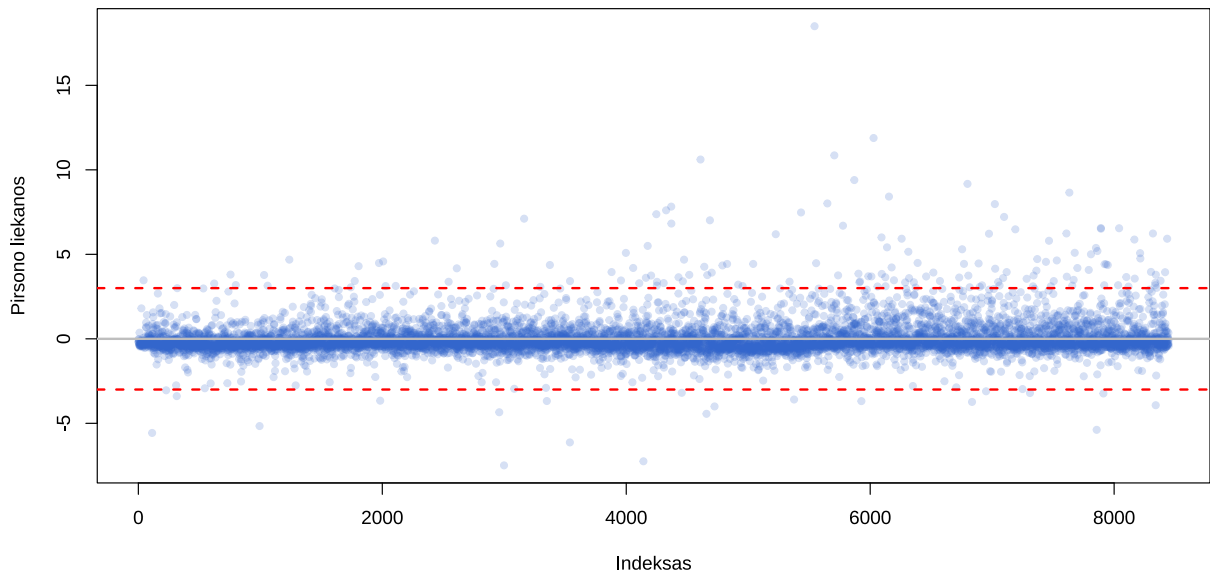
Lokatioji regresija: Pirsono liekanos
