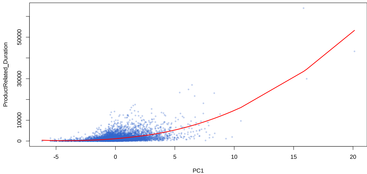
Lokatioji regresija: modelio tinkamumas
